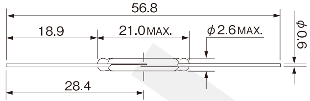
■外形寸法图(单位: mm) 外形尺寸图(单位: mm)
